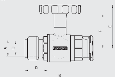
Pumpen-Kugelhahn TECTITE mit Schwerkraftbremse und rundem Thermometergriff
