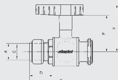
Pumpen-Kugelhahn TECTITE mit verlängertem Flügelgriff
