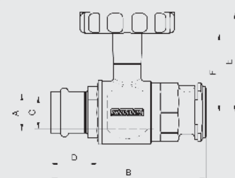
Pumpen-Kugelhahn PRESS mit Schwerkraftbremse und rundem Thermometergriff
