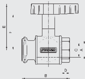
Pumpen-Kugelhahn mit verlängertem Flügelgriff
