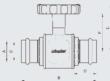
Muffen-Kugelhahn PRESS mit rundem Thermometergriff
