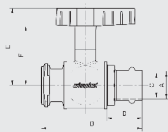
Pumpen-Kugelhahn PRESS mit verlängertem Flügelgriff
