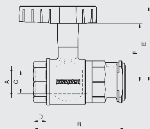
Pumpen-Kugelhahn mit Schwerkraftbremse und verlängertem Flügelgriff
