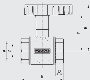
Muffen-Kugelhahn mit verlängertem Flügelgriff
